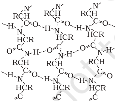
चित्र 14.2— प्रोटीन की \beta -प्लीटेड शीट संरचना
