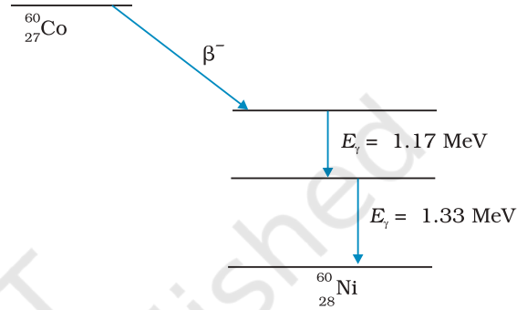
चित्र 13.4 ^{60}_{27}\text{Co} नाभिक के बीटा क्षय में उत्सर्जित \gamma -किरणों के उत्सर्जन को दर्शाने वाला ऊर्जा स्तर आरेख।
